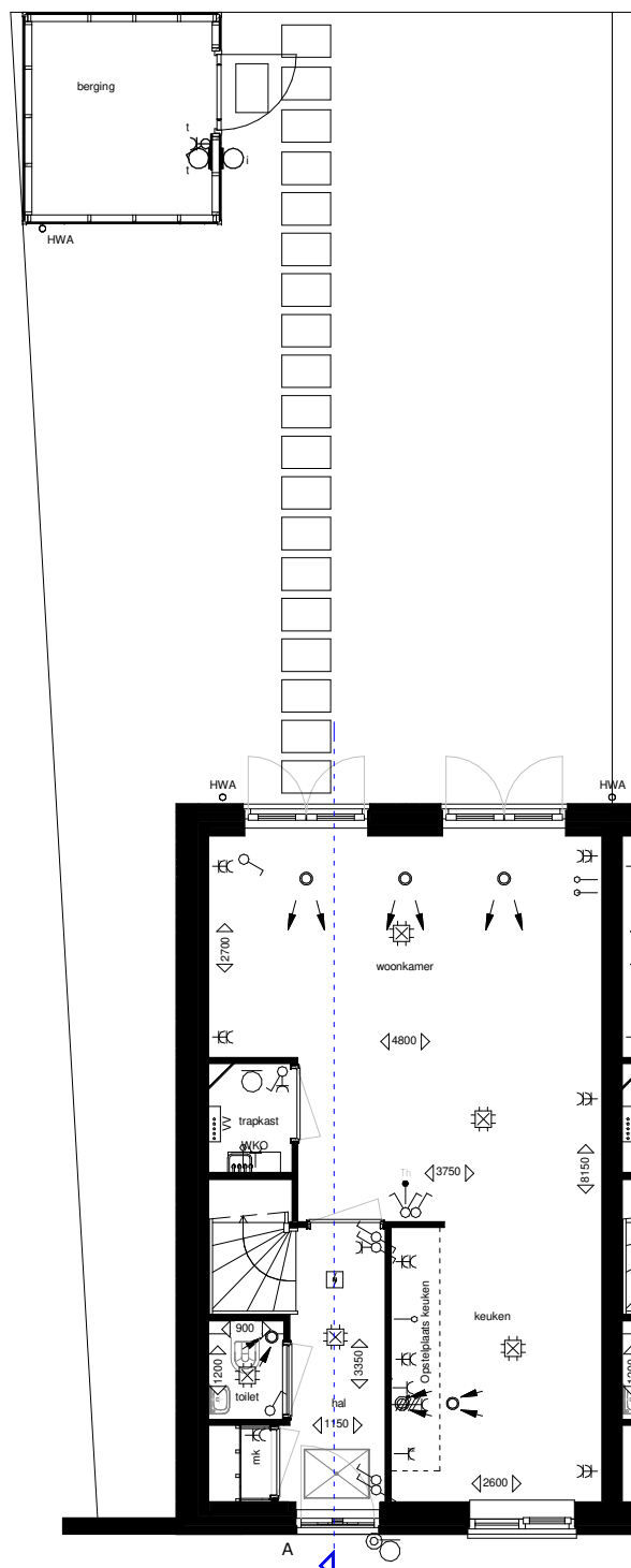
BEGANE GROND
